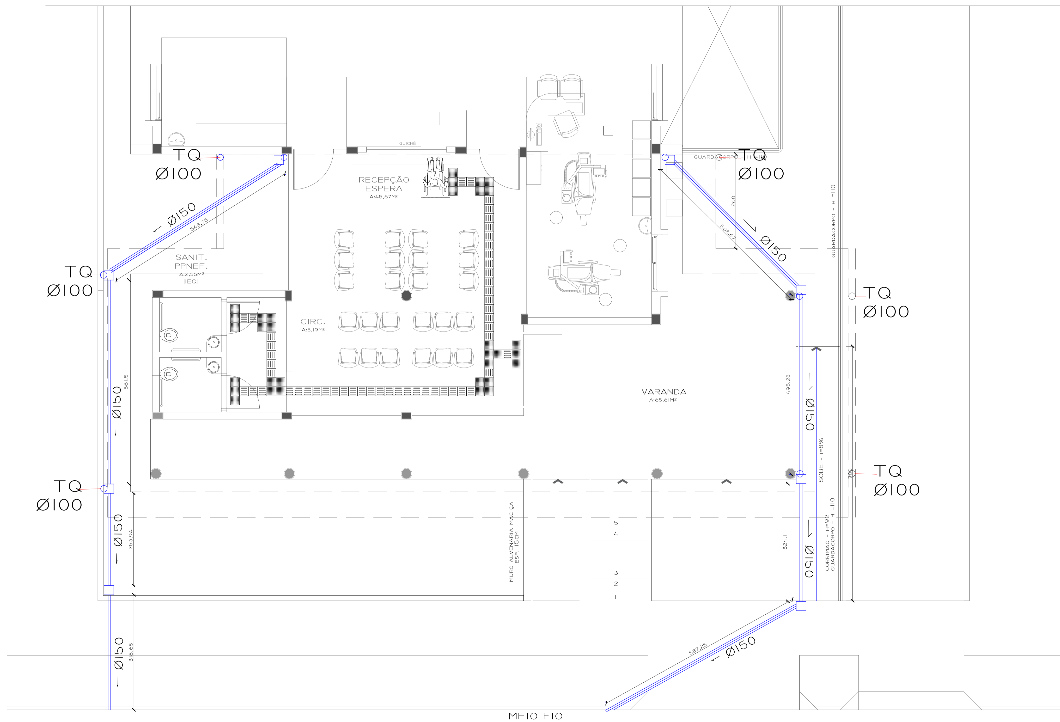
PLANTA DE DRENAGEM PLUVIAL ESCALA 1/50
