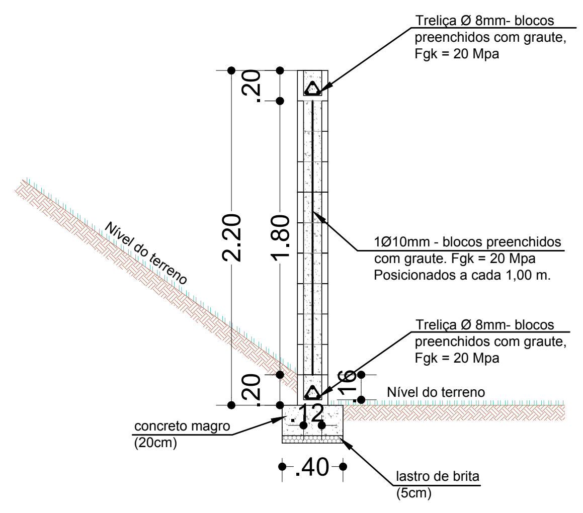
CORTE MURO ALVENARIA ESTRUTURAL ESCALA 1/25
