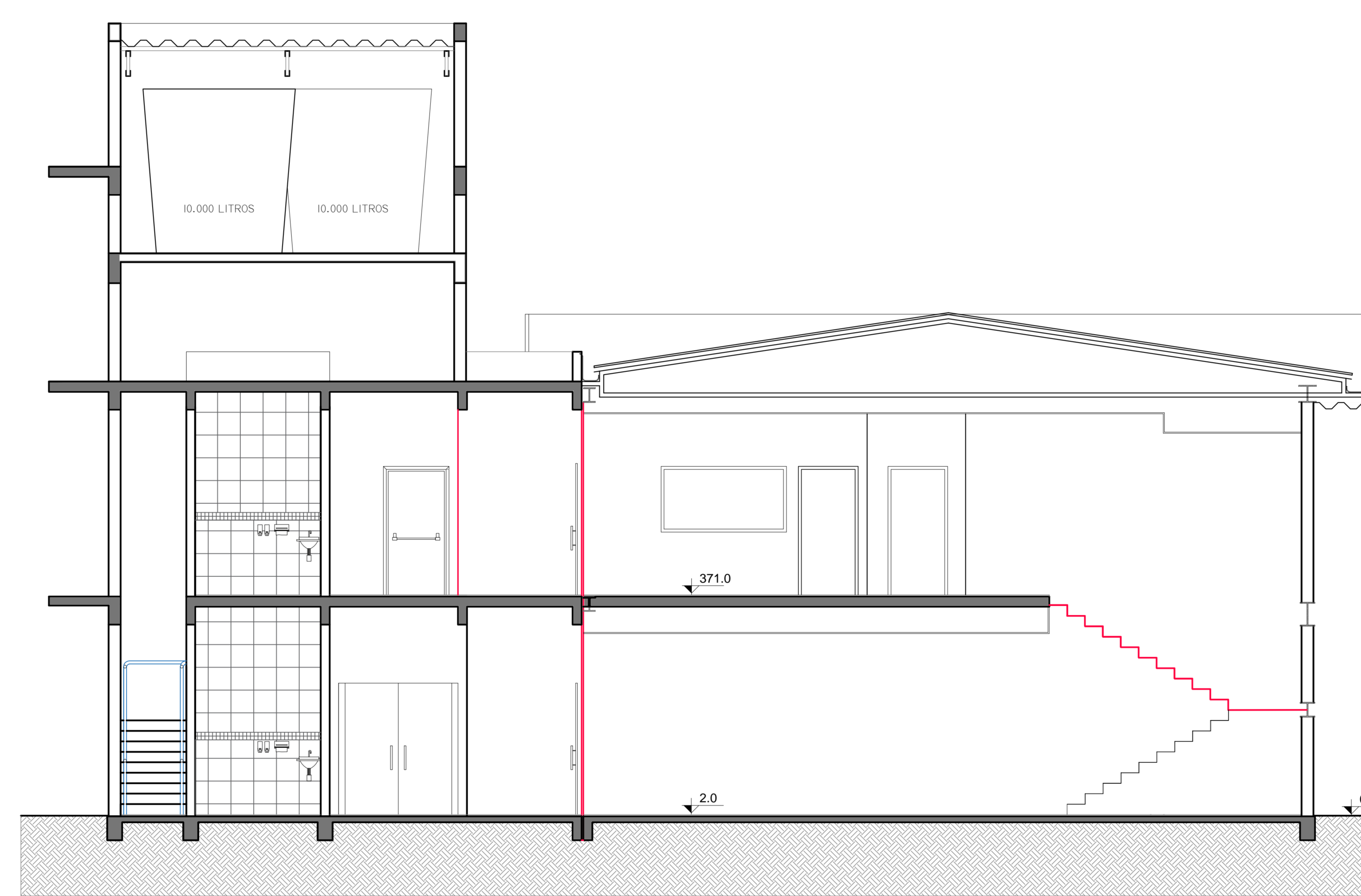
CORTE C-C
