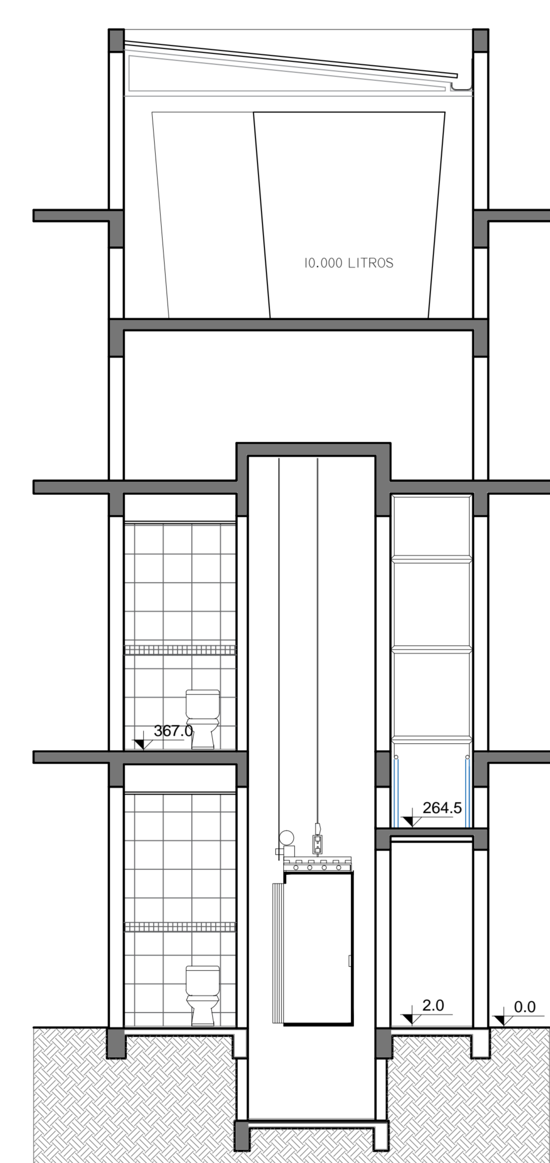
CORTE B-B
